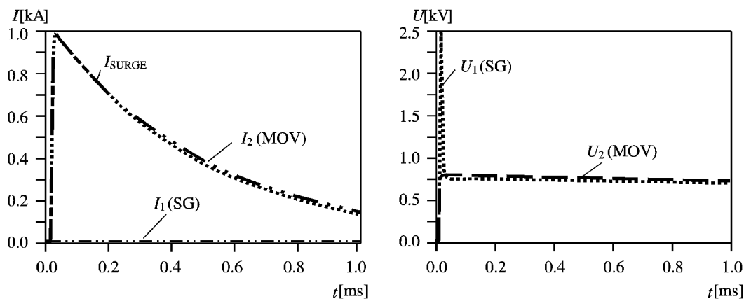
a) 电涌波形为 10/350 \mu\text{s} 时 SG 和 MOV 的电流和电压 (SPD1 未点火)
