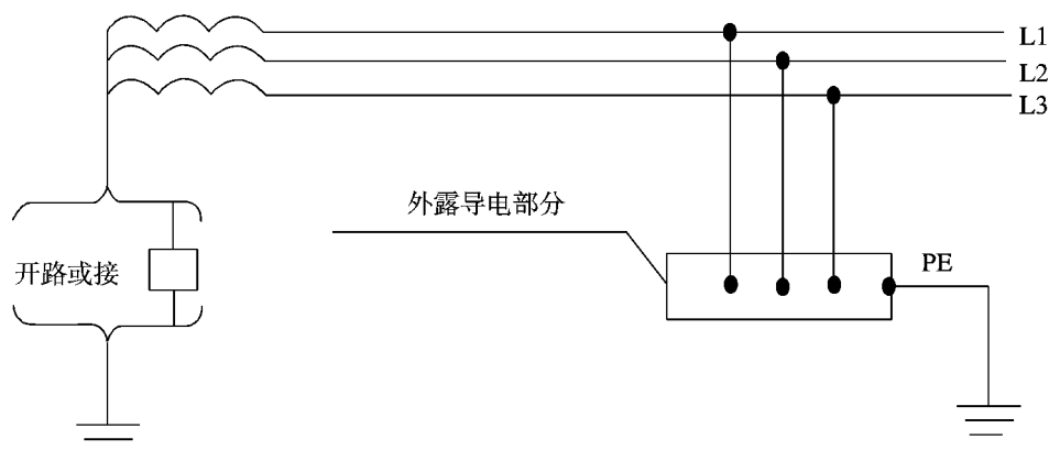
图 5 不配出中性线的 IT 系统
