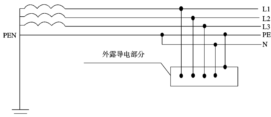
图 4 TN-C-S 系统
