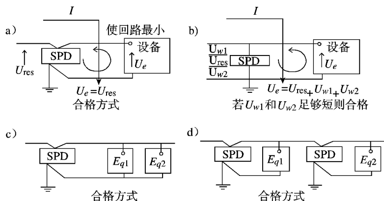
图 C.4 安装单端口 SPD 的常用方式
