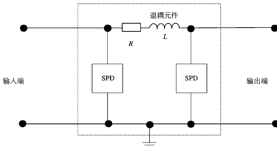
图 E.16 配合方案 IV (双口 SPD, 有若干限压元件并联组成)
