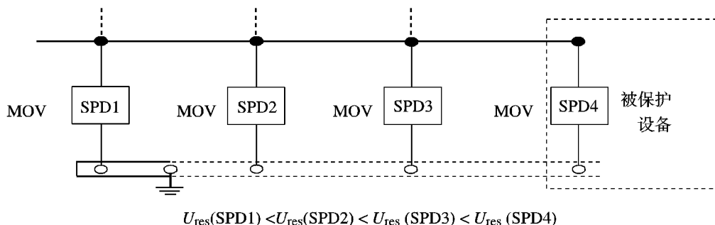
图 E.14 配合方案 II (限压型 SPD)
