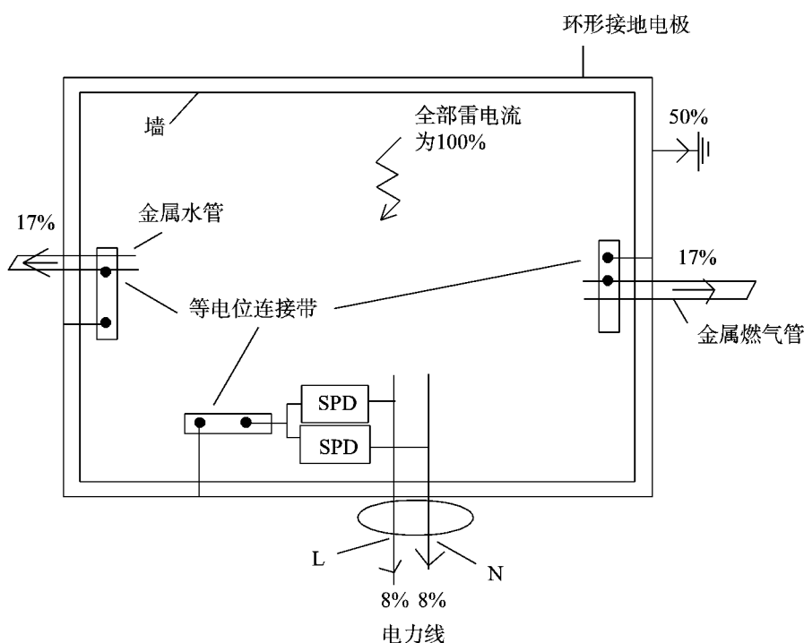
图 B.1 雷电流分配到内部设备的示例(TT 系统)
