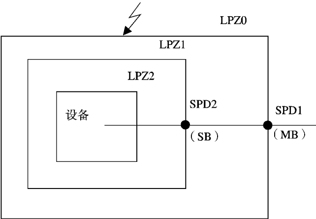
图 7 建筑物防雷区的划分和等电位连接位置示意图
