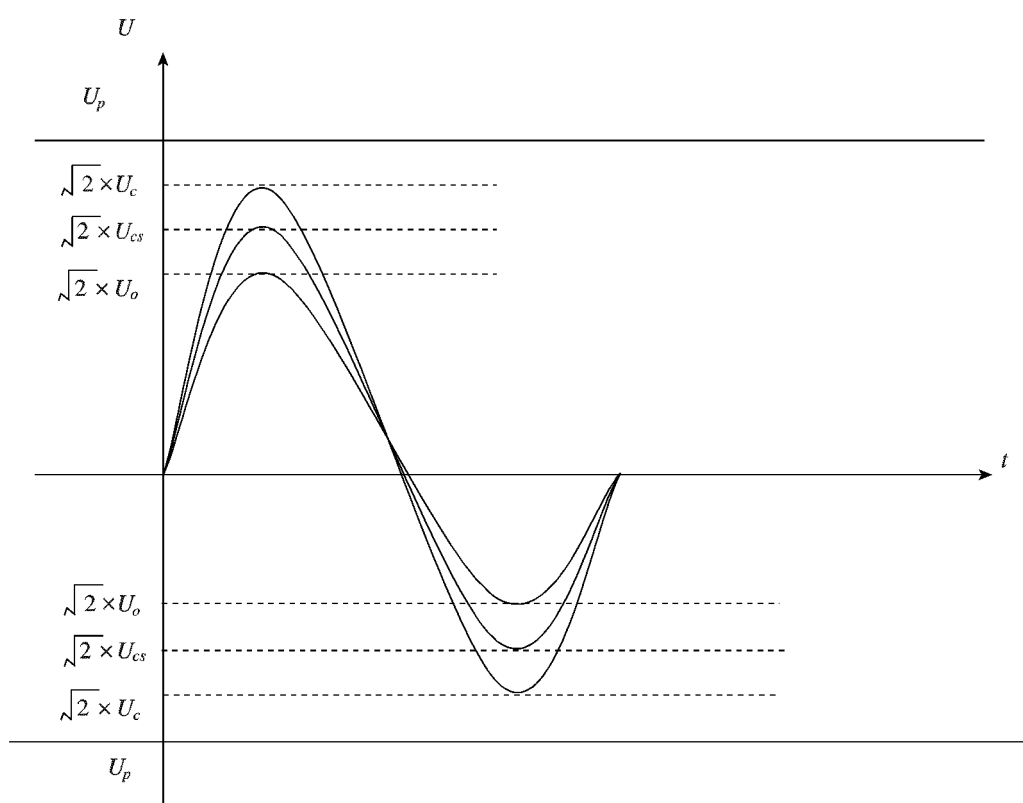
图 B.11 U_p 、 U_o 、 U_c 和 U_{cs} 之间的关系
