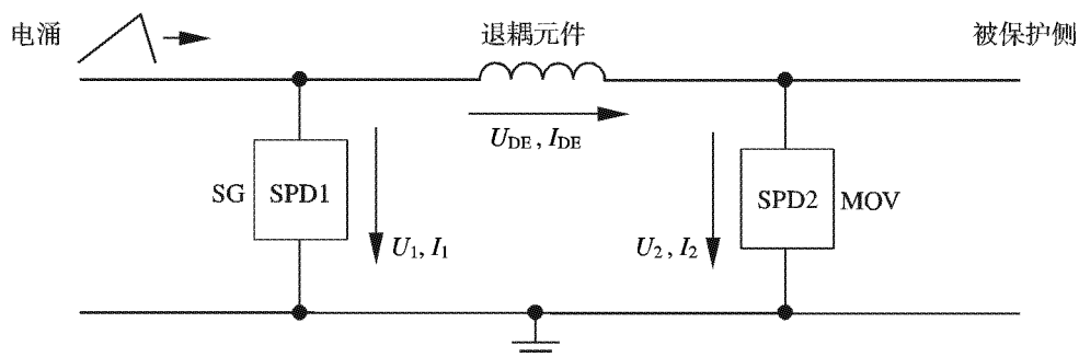
a) 有 SG 和 MOV 的电路
