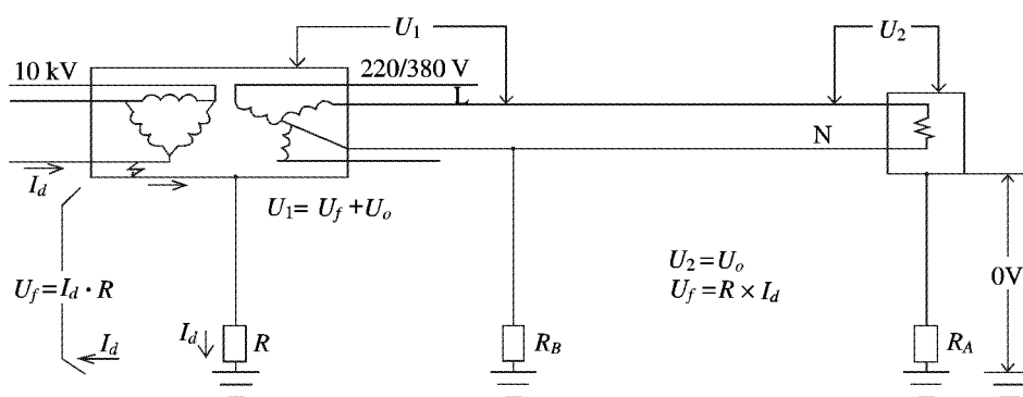
图 B.9 TT 系统(高压保护地与低压系统地为分开的接地极)
