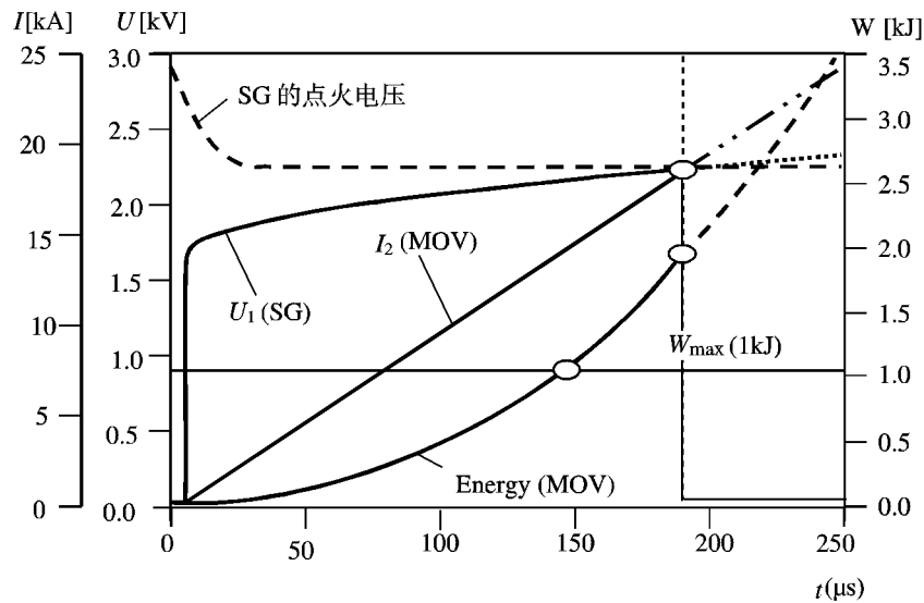
b) L_{DE} = 10 \mu\text{H} 时的电流/电压/能量特性: 电涌为 0.1 \text{ kA}/\mu\text{s} 时未达到能量配合
