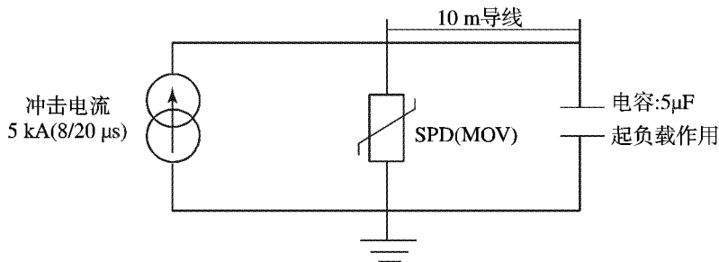
图 E.2 MOV 和被保护设备之间可能产生的振荡
