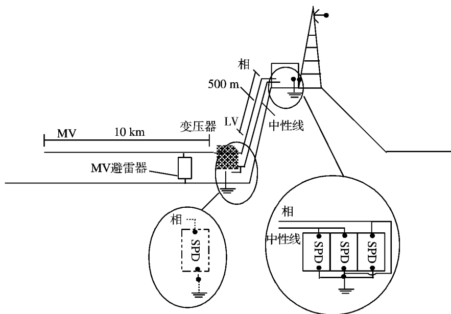
图 D.3 RBS 的系统组成
