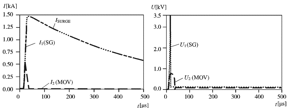
b) 电涌波形为 10/350 \mu\text{s} 时 SG 和 MOV 的电流和电压 (SPD1 点火)
