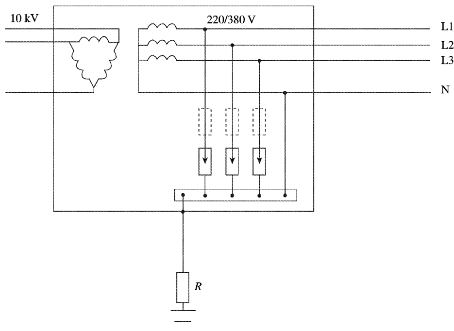
图 C.1 10 kV 的保护接地与 LV 系统的中性线接地共用一个接地极的变电所内 TT 系统和 TN 系统 SPD 的安装
