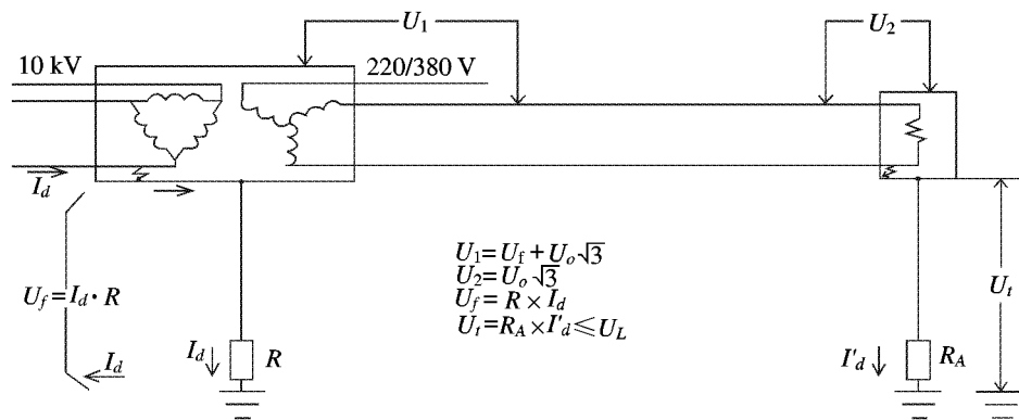
图 B.10 IT 系统(高压系统与低压系统同时出现接地故障的情况)
