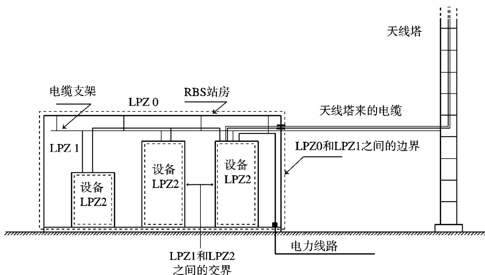
图 D.4 RBS 的防雷区 (LPZ) 划分
