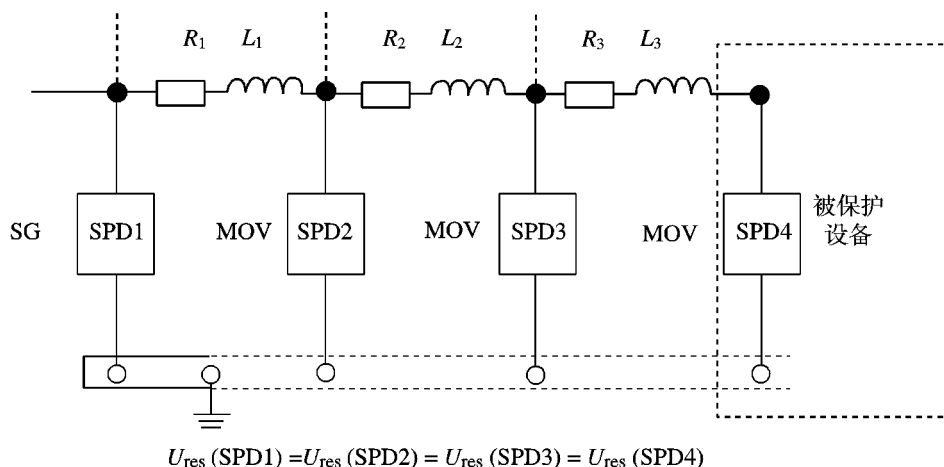
图 E.15 配合方案 III (电压开关型和限压型 SPD)
