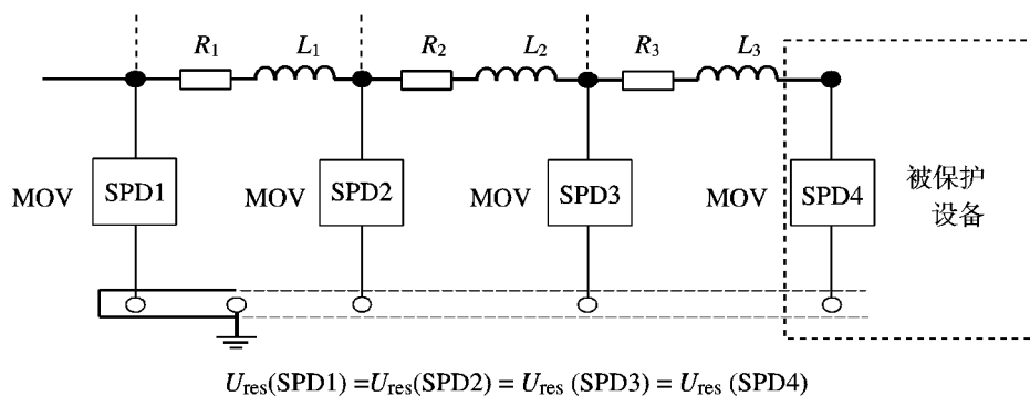
图 E.13 配合方案 I (限压型 SPD)
