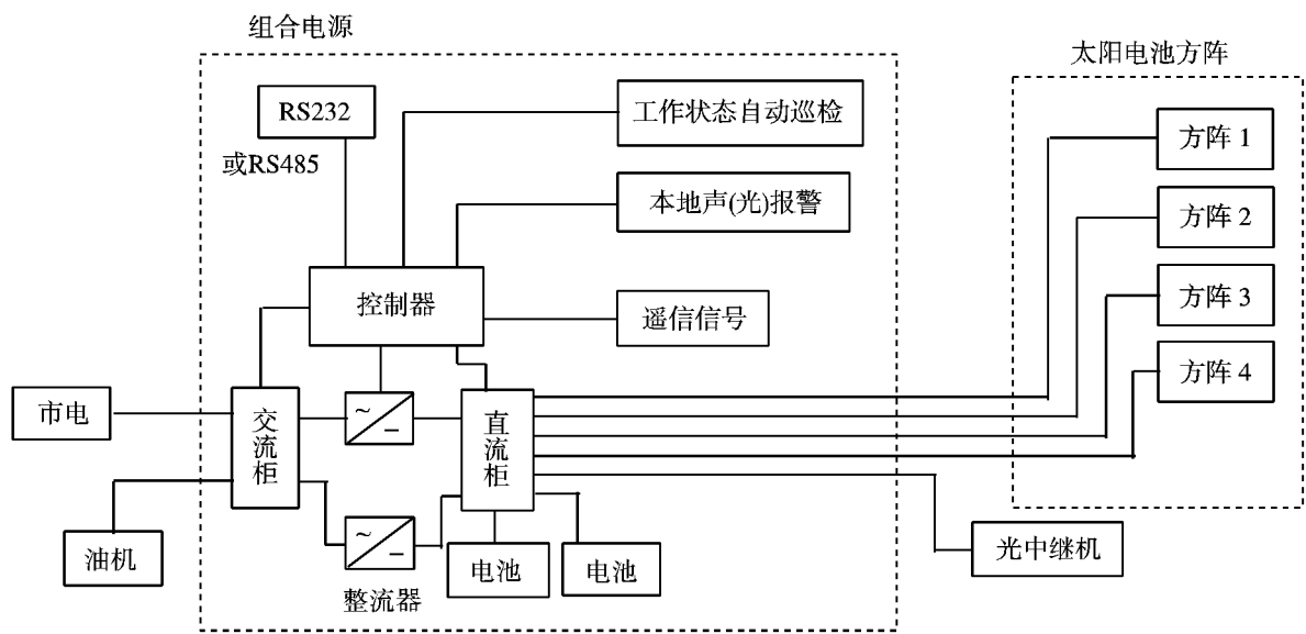
图 D.5 市电(油机)与太阳能发电系统组成示意图
