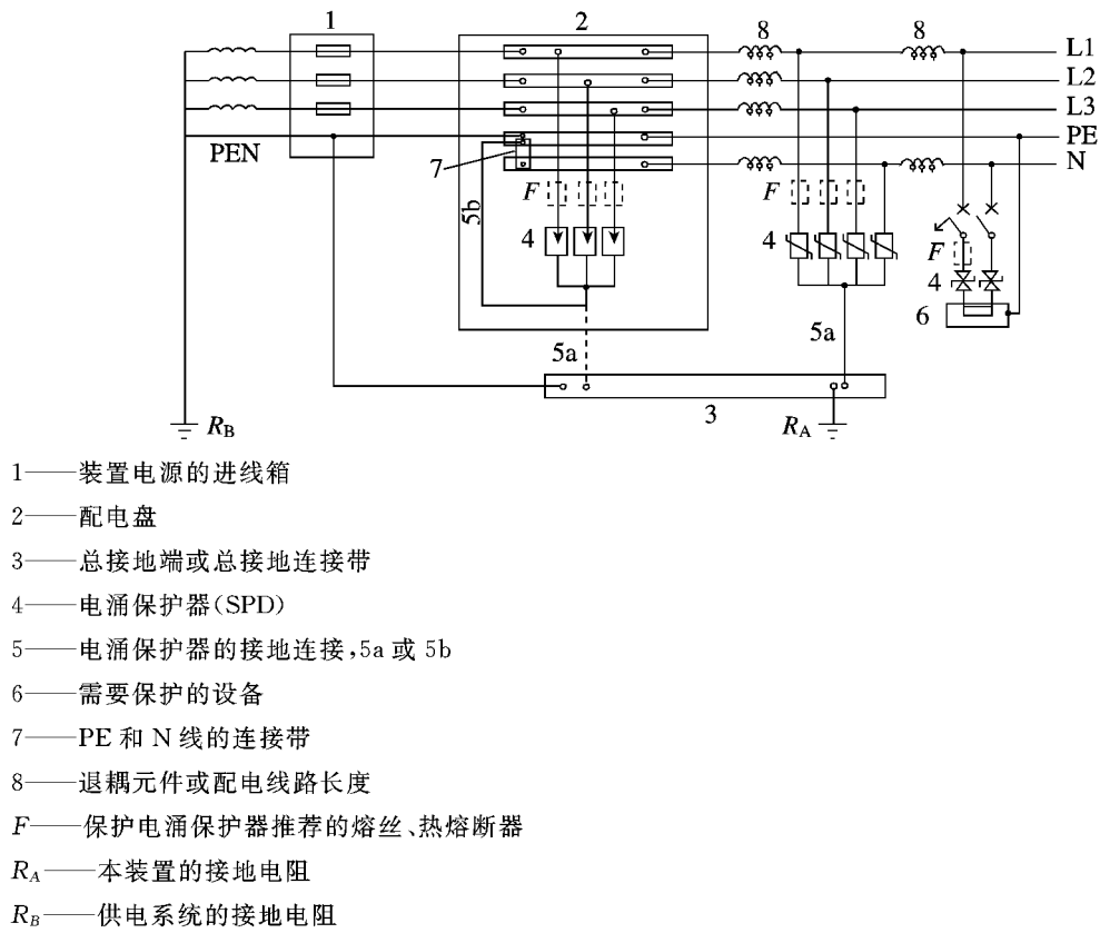
图 14 在 TN-C-S 系统中 SPD 的安装示例
