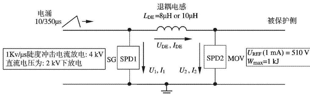
a) 电涌波形为 10/350 \mu s 时能量配合的电路图示例
