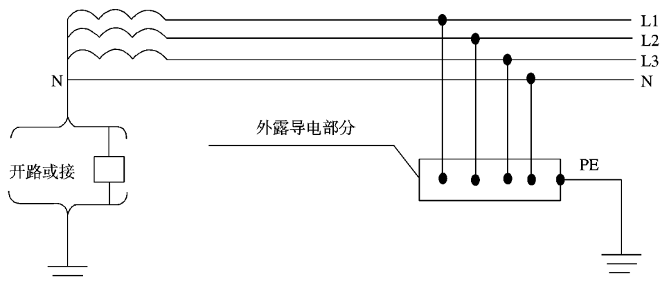
图 6 配出中性线的 IT 系统
