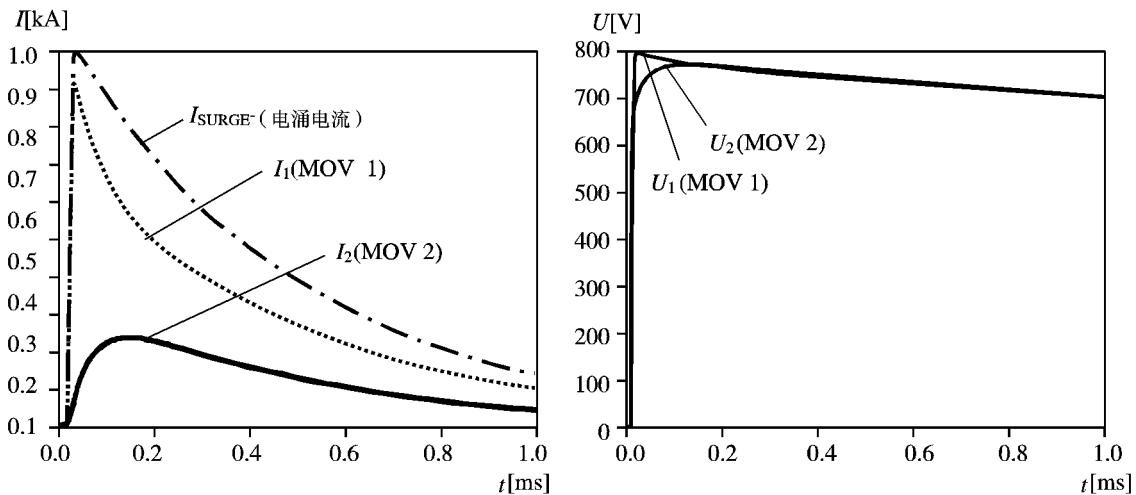
b) 电涌波形为 10/350 \mu s 时 MOV 1 和 MOV 2 的电流和电压
