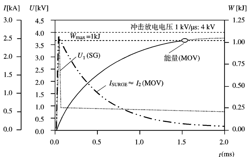
b) L_{DE} = 8 \mu\text{H} 时的电流/电压/能量特性: 电涌波形为 10/350 \mu\text{s} 时未达到能量配合 (SG 未点火)
