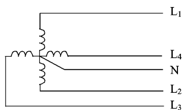
图 A.4 两相五线系统
