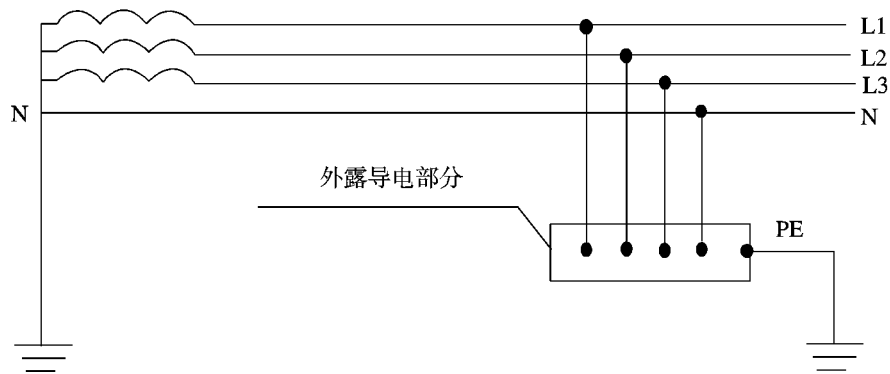
图 1 TT 系统
