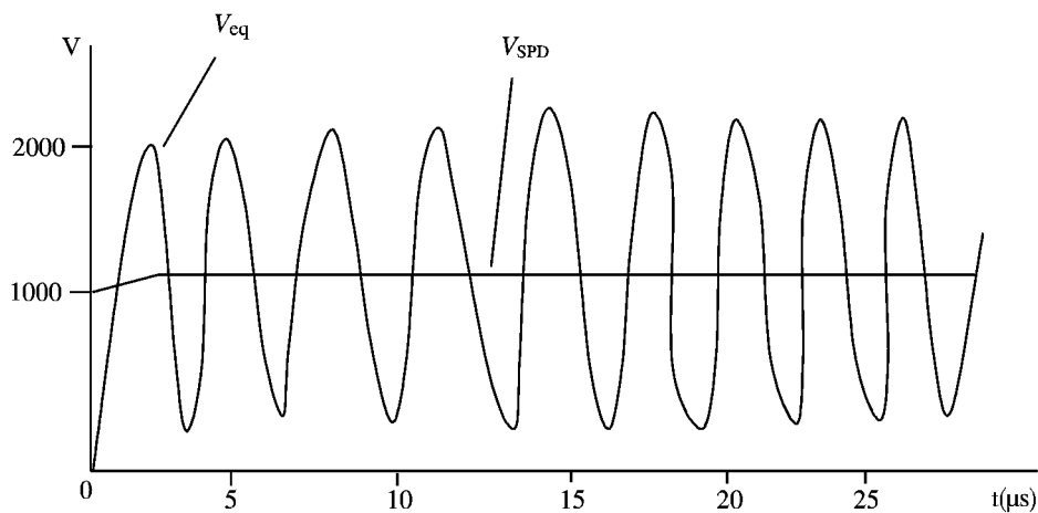
图 E.2 MOV 和被保护设备之间可能产生的振荡
