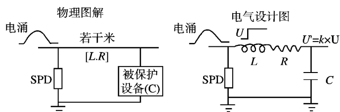
图 E.1 SPD 后端电压翻倍的图解
