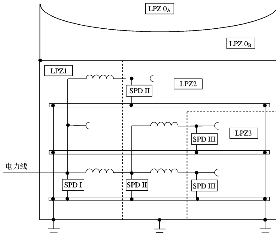
图 E.4 在电气系统中 SPD 的应用示例
