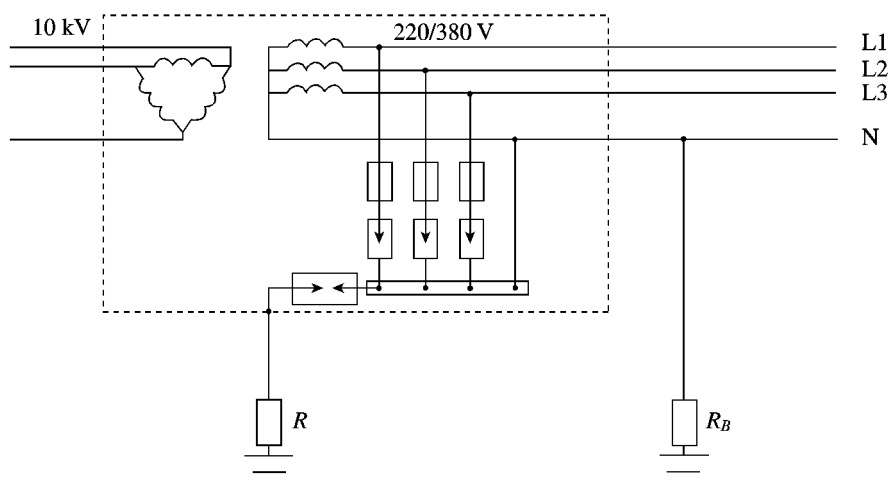
图 C.2 10 kV 的保护接地与 LV 系统的中性线接地为分开接地极的变电所内 TT 系统和 TN 系统 SPD 的安装
