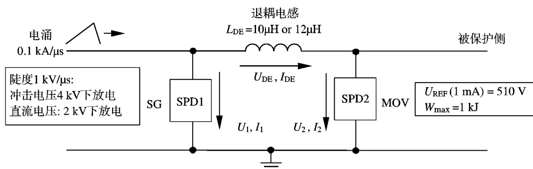
a) 电涌为 0.1 kA/ \mu\text{s} 时能量配合的电路图
