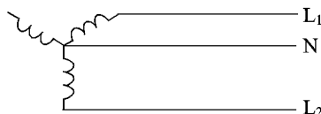
图 A.3 两相三线系统
