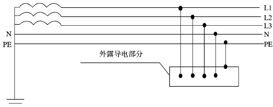
图 3 TN—S 系统
