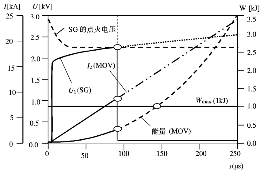
c) L_{DE} = 12 \mu\text{H} 时的电流/电压/能量特性: 电涌为 0.1 \text{ kA}/\mu\text{s} 时达到能量配合
