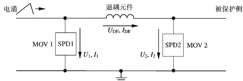
a) 有 MOV 1 和 MOV 2 配合的电路
