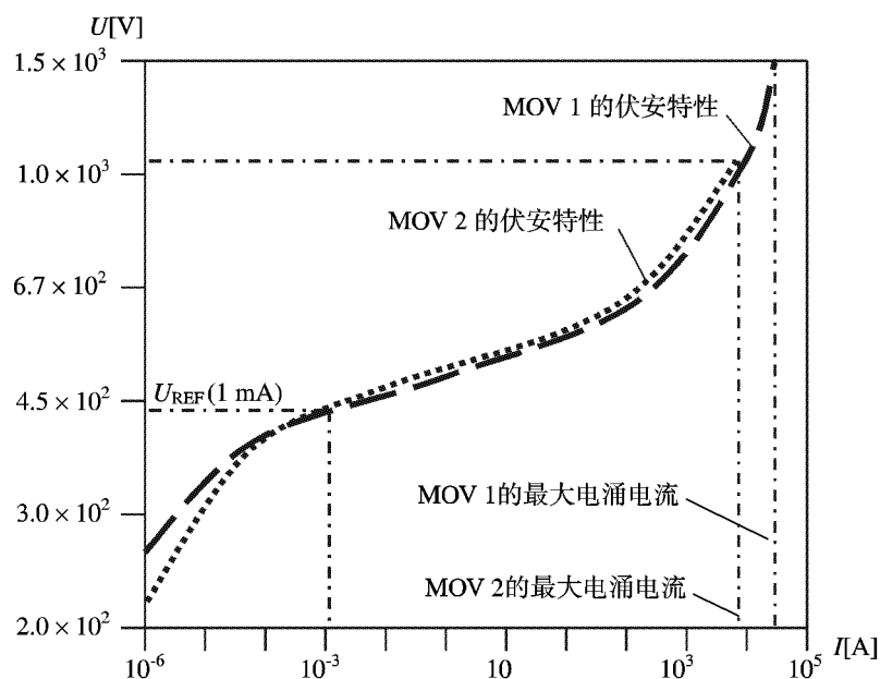
a) MOV 1 和 MOV 2 的伏安特性
