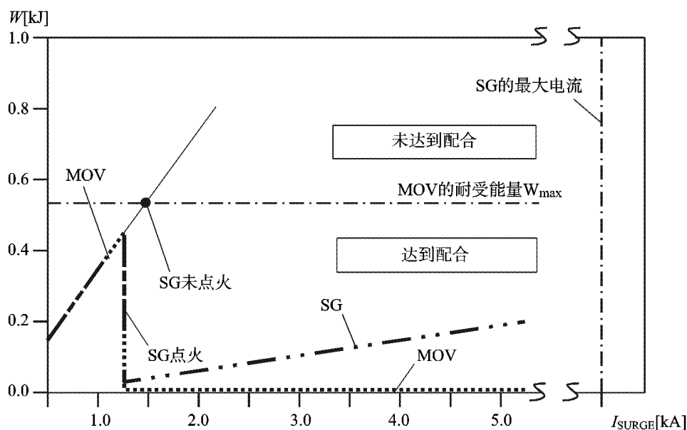
b) SG 和 MOV 的能量配合原理
