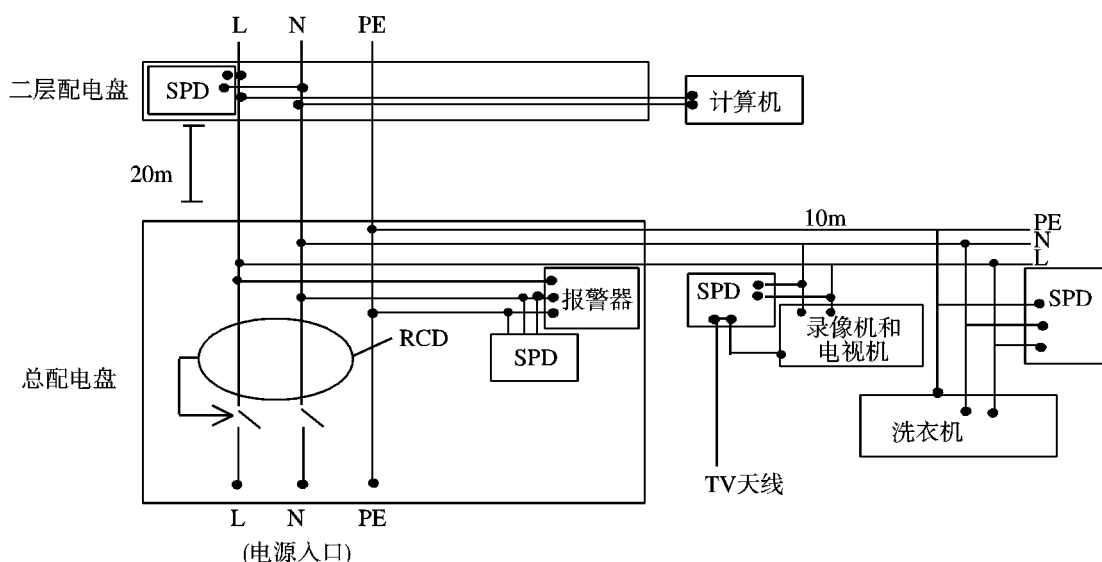
图 D.2 SPD 安装位置示意图
