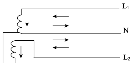
图 A.2 单相三线系统
