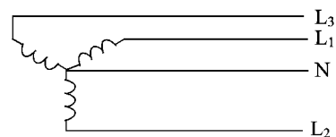
图 A.6 三相四线系统
