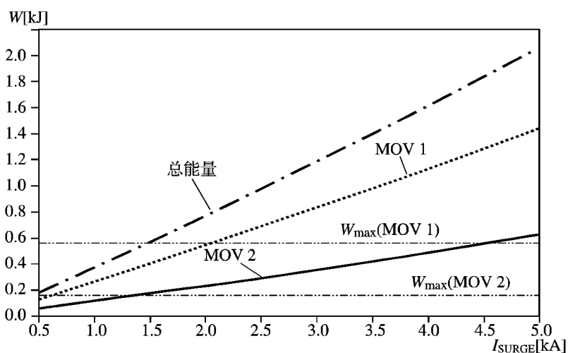
b) MOV 1 和 MOV 2 的能量配合原理
