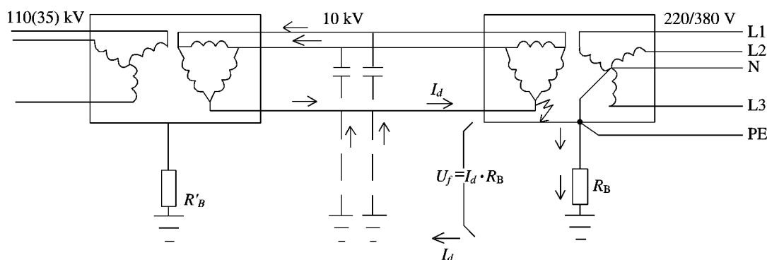
图 B.3 10 kV 不接地系统内 I_d 值和 U_f 值均很小
