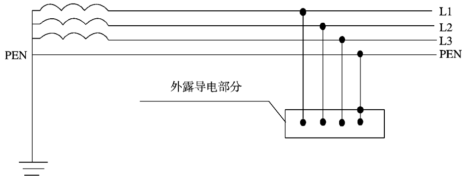
图 2 TN—C 系统
