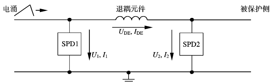
图 E.5 SPD 能量配合的基本模型
