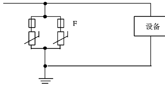
c) 兼顾供电连续性和保护连续性
