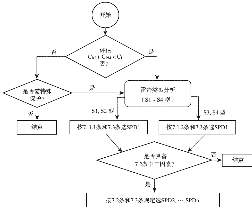
图9 选择 SPD 的流程图
