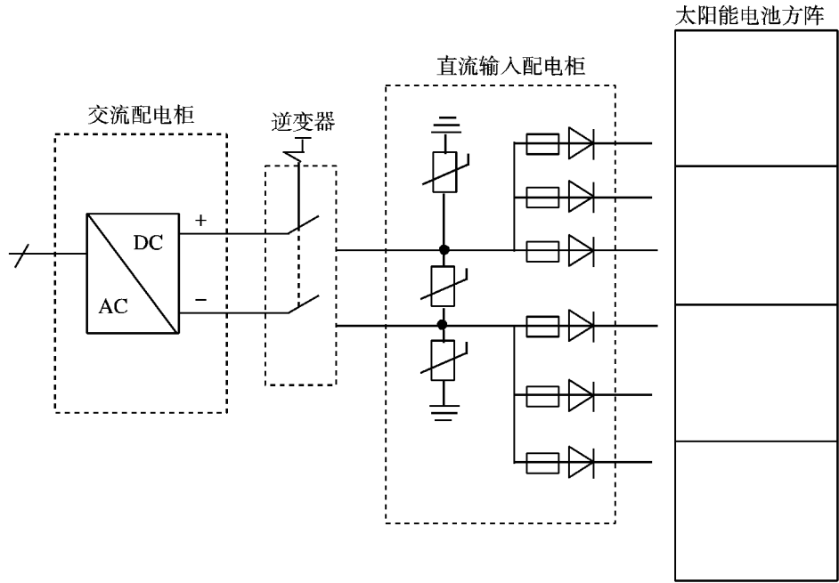
图 D.6 SPD 在太阳能发电系统中的安装示例
