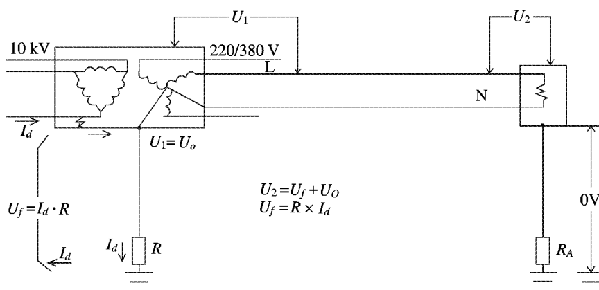
图 B.8 TT 系统(高压保护地与低压系统地共用一个接地极)
