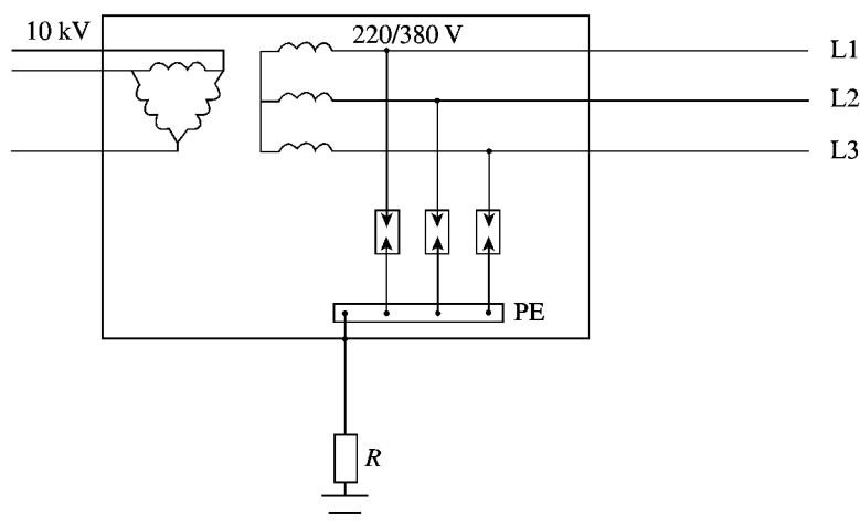
图 C.3 采用 10 kV 经小电阻接地系统的变电所内，IT 系统 SPD 的安装
