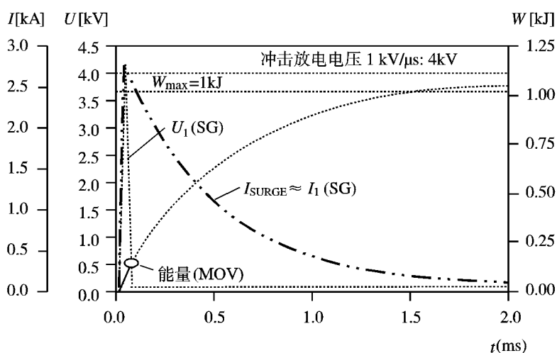
c) L_{DE} = 10 \mu\text{H} 时的电流/电压/能量特性: 电涌波形为 10/350 \mu\text{s} 时达到能量配合 (SG 点火)
