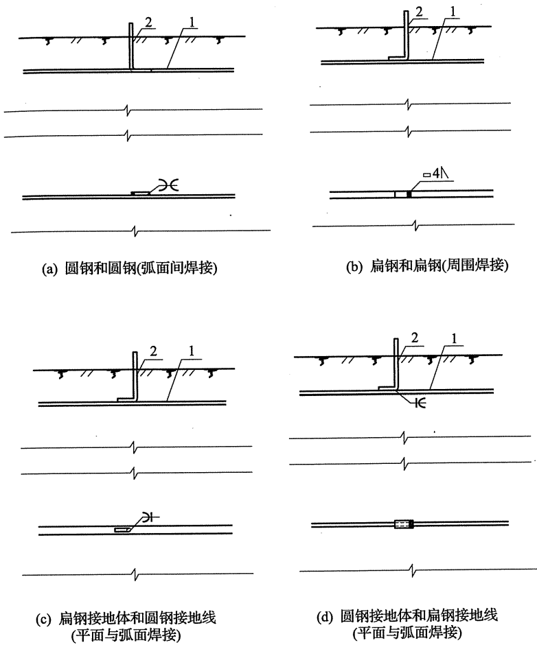
图 C.1.2-1 使用圆钢、扁钢的人工水平接地体施工
