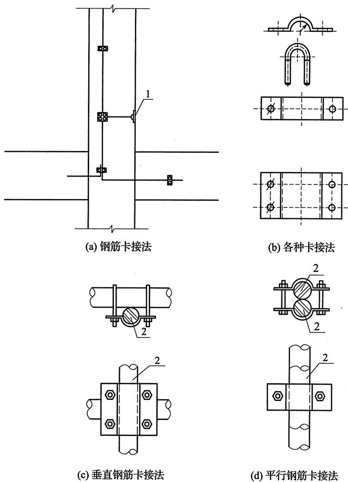
图 C.2.1-1 混凝土内钢筋之间的卡接
