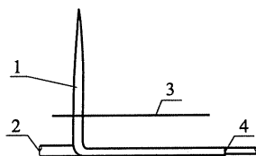
图 C. 3. 4 短接闪杆的施工
