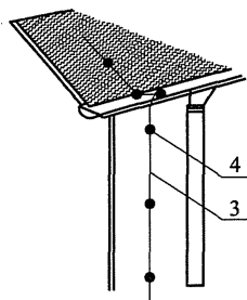
(b) 与接闪带及屋檐排水沟连接的引下线的安装
