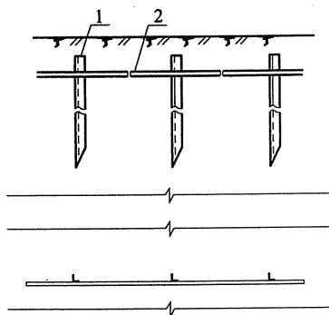
(a) 接地体安装
