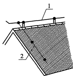
(a) 坡屋顶上接闪器的安装
