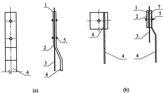
图 C. 2. 2 金属屋面与引下线连接
