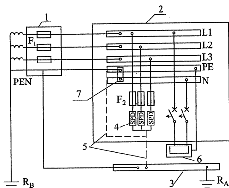
图 C. 4. 1 TN 系统中的 SPD
