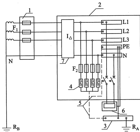
图 C. 4. 2-1 TT 系统中 SPD 安装在剩余电流保护器的负荷侧
