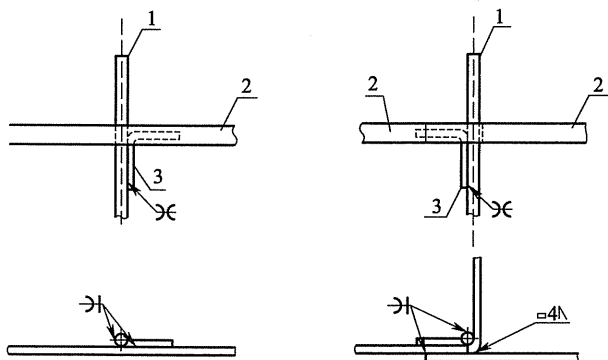
(c) 圆钢垂直接地体与扁钢水平接地体的连接
