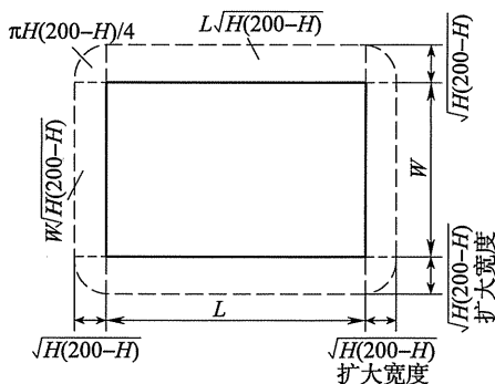
图 A. 0. 3 农村民居的等效面积
