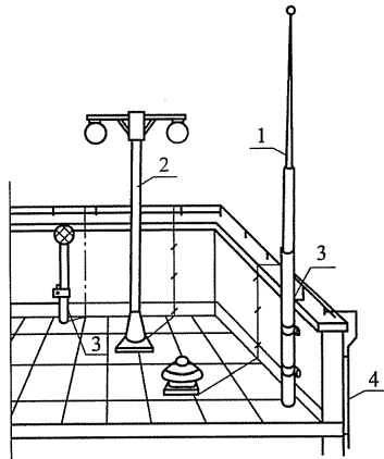
图 C.3.6 屋顶透气管、金属灯杆、 旗杆防雷装置安装 1—金属旗杆;2—金属灯柱; 3—焊接或卡接;4—引下线
