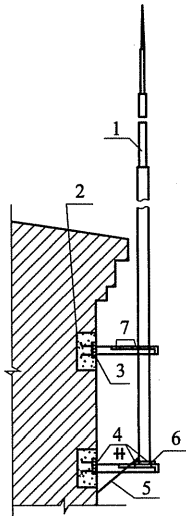
图 C.3.5 接闪杆在侧墙上安装 1—接闪杆;2—钢筋混凝土梁;3—预埋钢板; 4—焊接;5—引下线;6—支持板;7—支架
