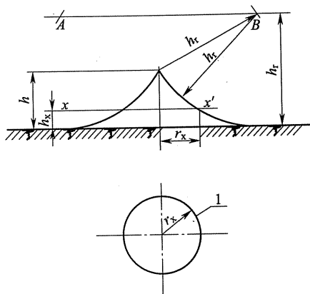
图 B.0.1 单支接闪杆的保护范围
