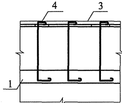
(d) 多根竖筋(剖面)
