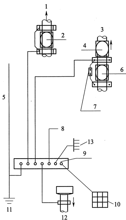
图 C. 5. 1 总等电位连接示意
