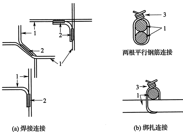
图 C. 2. 1-2 混凝土内钢筋之间的连接
